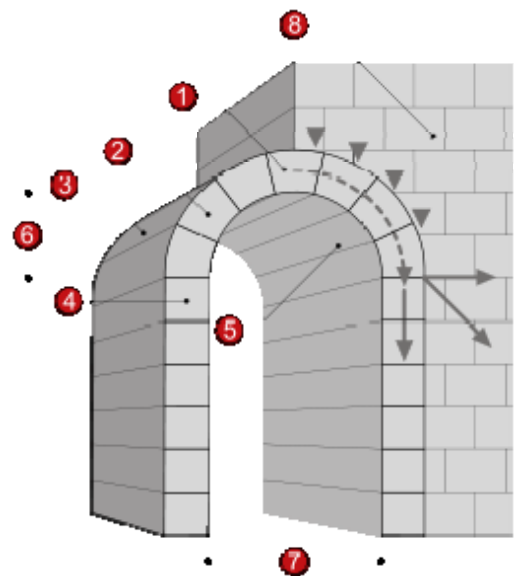
Nomenclatura della volta a botte: (1) chiave di volta; (2) cuneo; (3) estradosso; (4) piedritto; (5) intradosso; (6) freccia; (7) corda; (8) rinfiacco.
